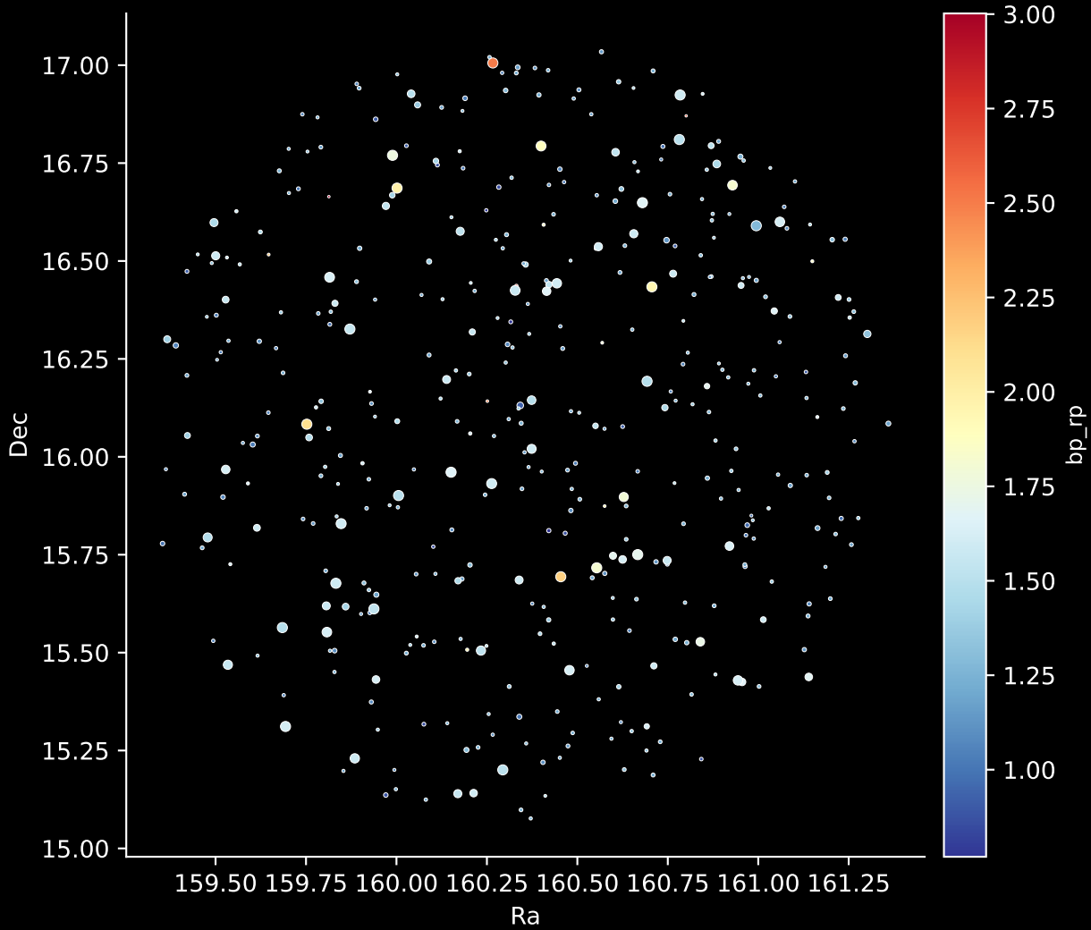
GALAH DR4 Field: [6591] Stars: 424
