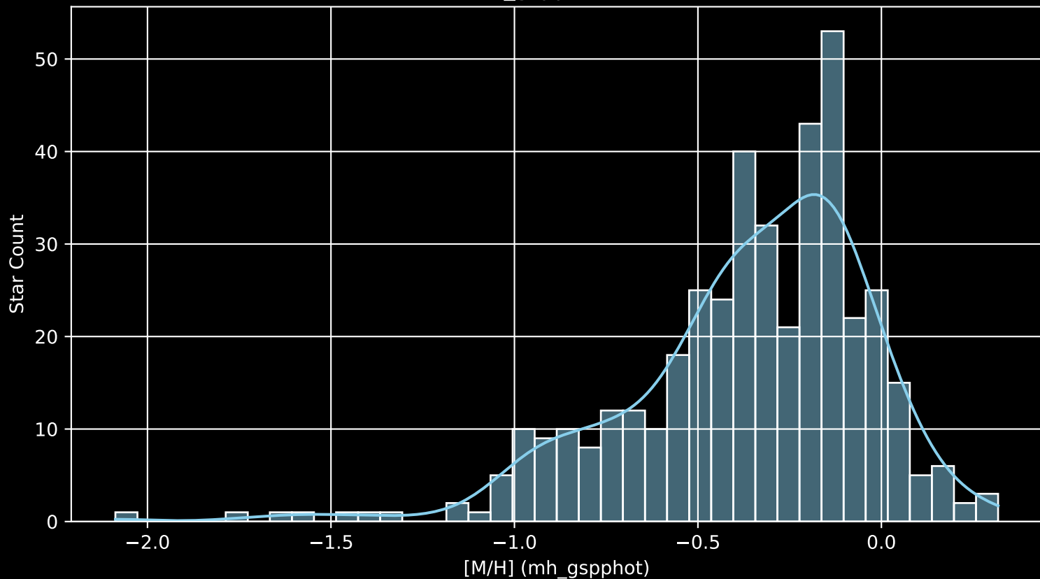
GALAH DR4 Field: [6591] [M/H] (mh_gspphot) (n= 420)
