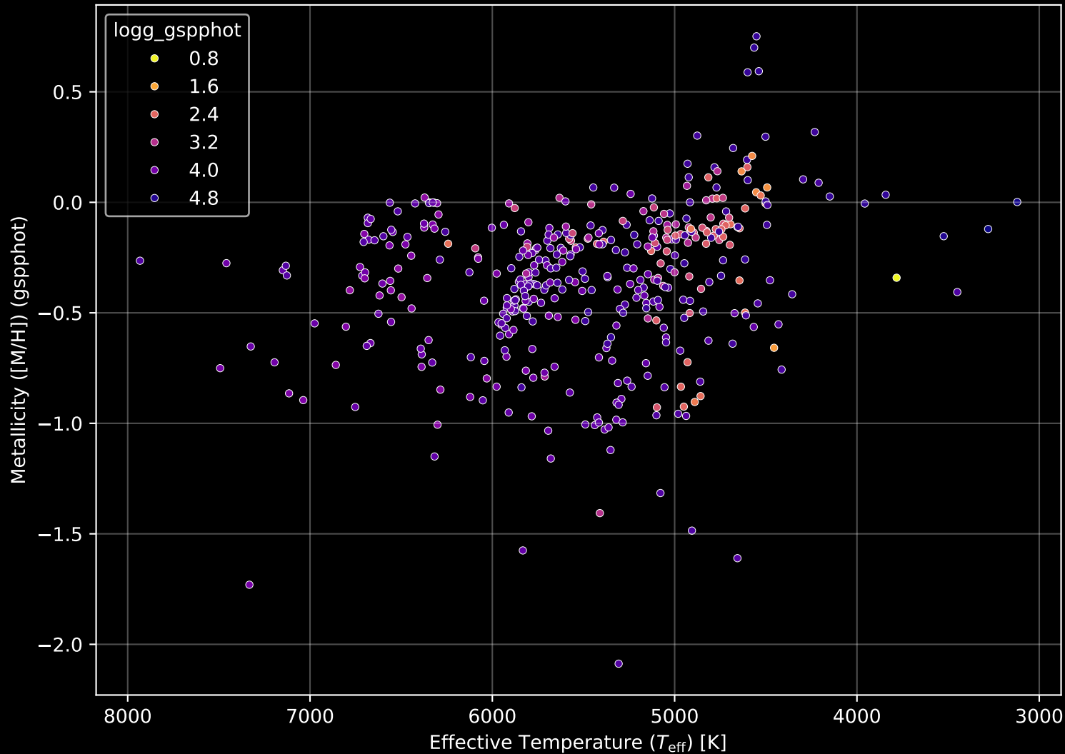
GALAH DR4 Field: [6591] Stellar Population Parameters (n= 424)
